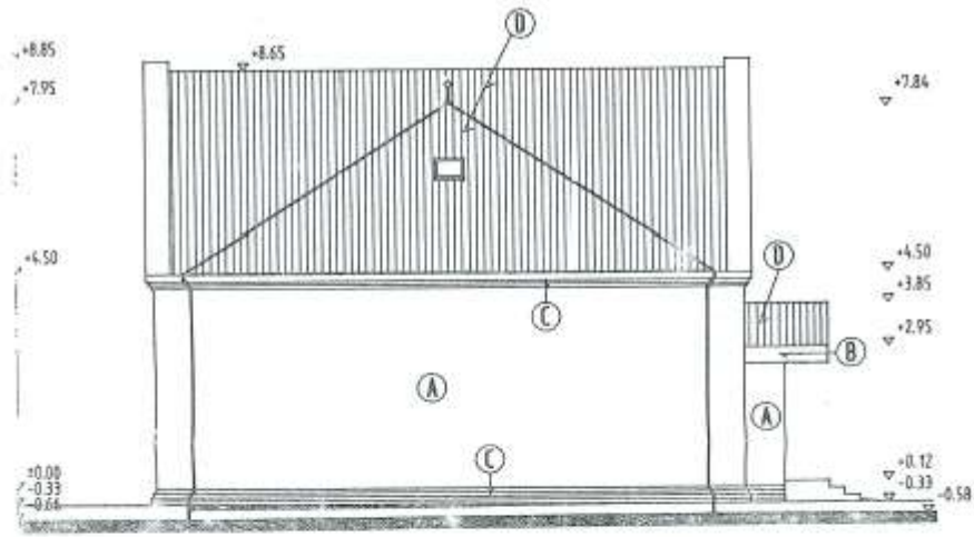
POHLED SEVEROVÝCHODNÝ
